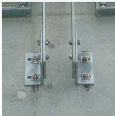
Canales dentados instalados verticalmente
