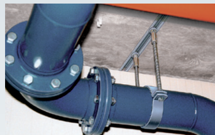
Instalación de tuberías
