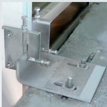
Sistema sobre losa (TOS)
