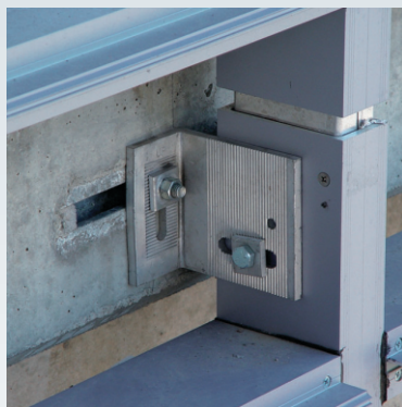
Sistema en canto de losa (FOS)
